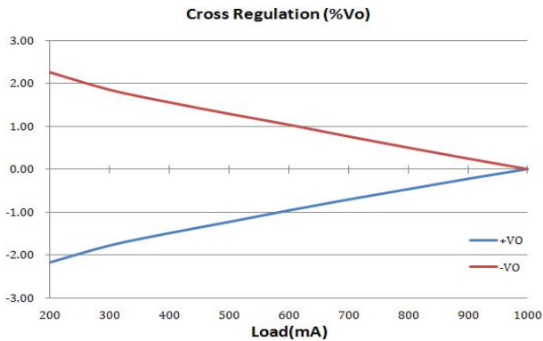
+Vo=1000mA, -Vo=200~1000mA
