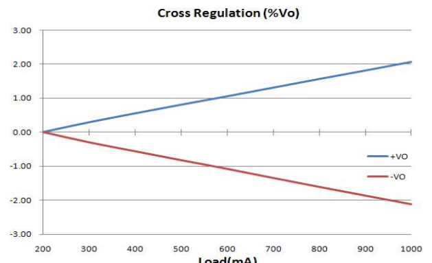
+Vo=200mA, -Vo=200~1000mA
