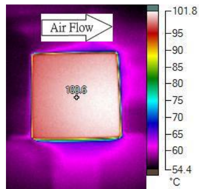
24Vin, 满载, 200LFM, 环温=49°C
