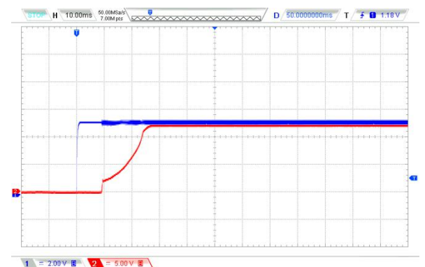
Vin=48VDC @100%Load
