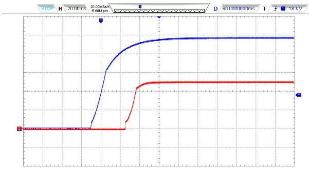
Vin=48VDC @100%Load
