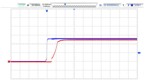
Vin=48VDC @100%Load
