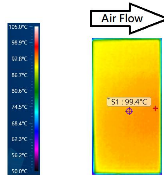
12Vin, 满载, 200LFM, 环温=57.4°C
