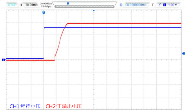
启动波形 ---程控启动
