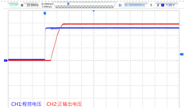
Vin=12VDC @100%Load +1500uF/EC
