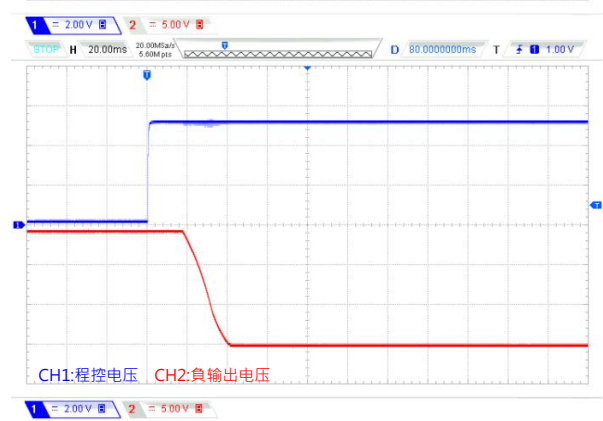
Vin=12VDC @100%Load +1500uF/EC
