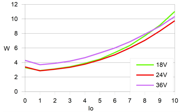
功耗曲线
