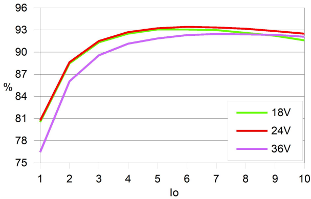
效率曲线
