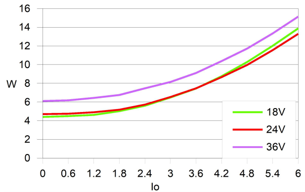
功耗曲线
