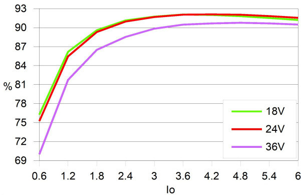
效率曲线
