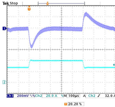
动态负载波形 ( V_{IN} : 24V, Load: 75%/50% @ 2.5A/µs)
