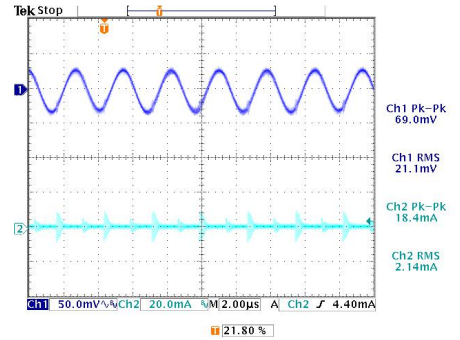
输入电流纹波/输出电压纹波噪声 ( V_{IN} : 24V, Load: 100%, L_{in} =10µH / C_{in} =470µF)
